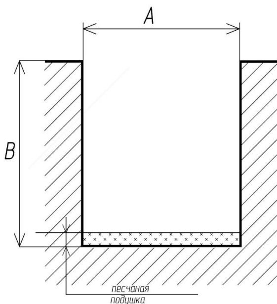
Подготовка котлована
